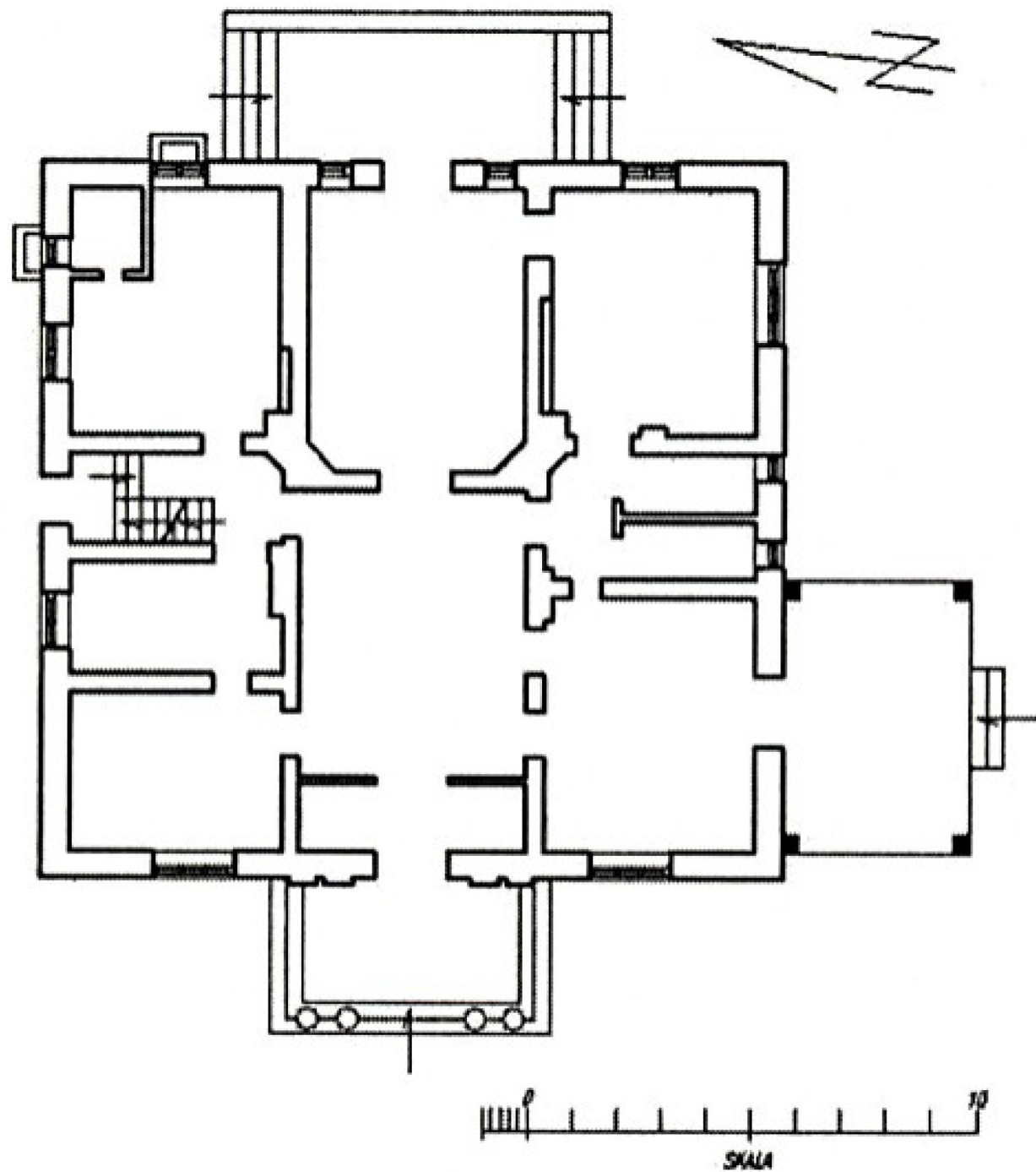
Dwór – rzut parteru. Oprac. Ewa R. Kowalewska
